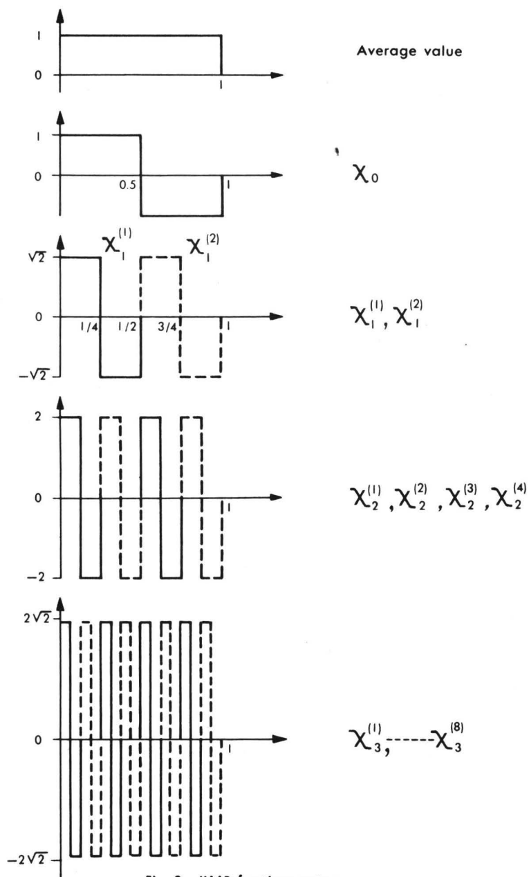
Fig. 2 - HAAR functions system
